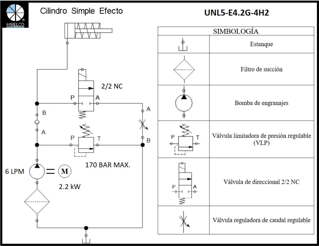
Imagen 3: Circuito hidráulico y tabla de simbología
