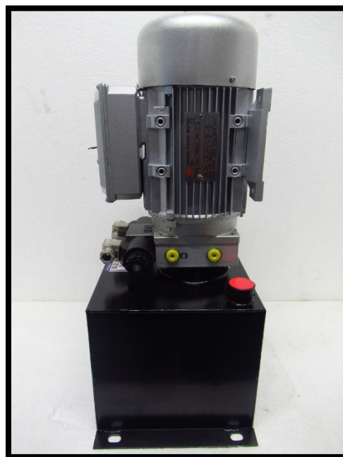
Imagen 1: Imágenes de Central hidráulica de doble efecto 220 VAC
